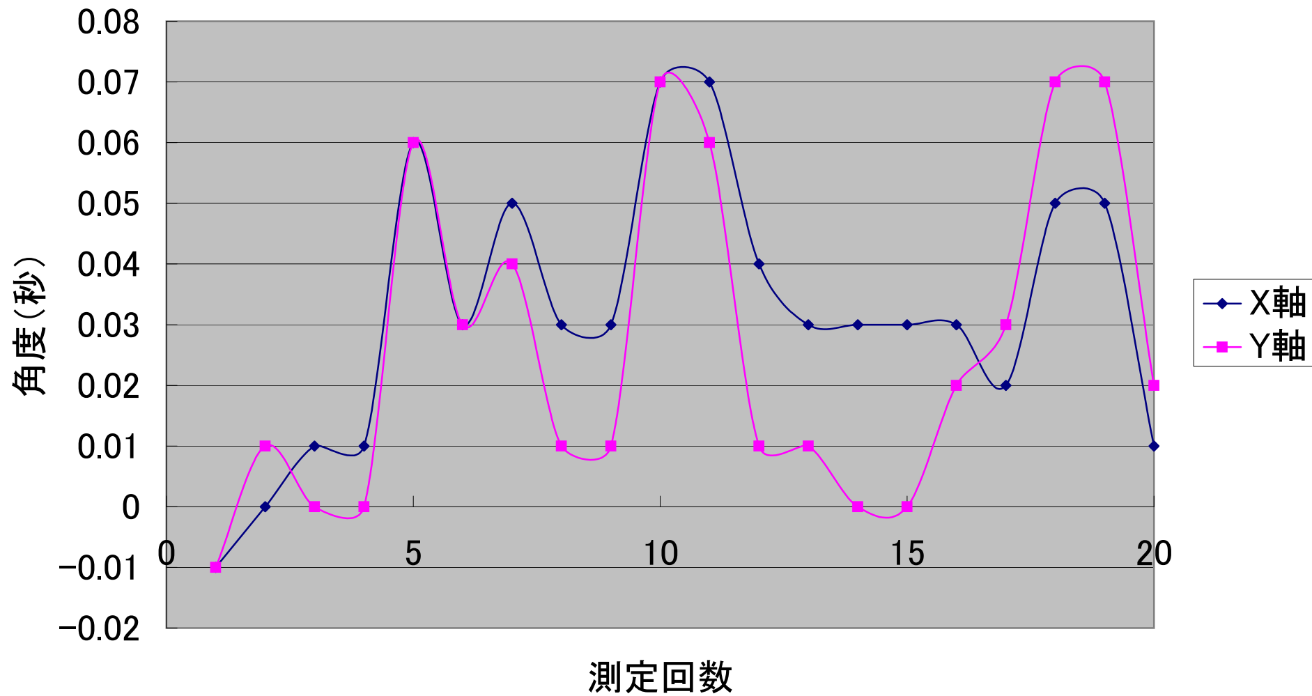
WD150 10秒ごとに20回測定安定性 (空気揺らぎ含む)
